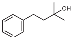
Benzenepropanol,1,1-dimethyl-
